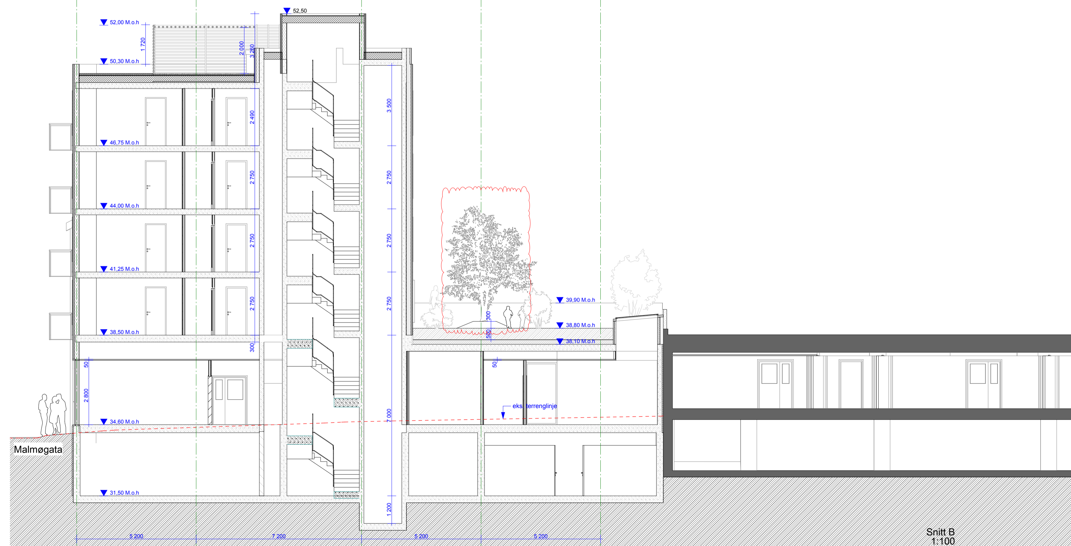
Snitt A 1:100
