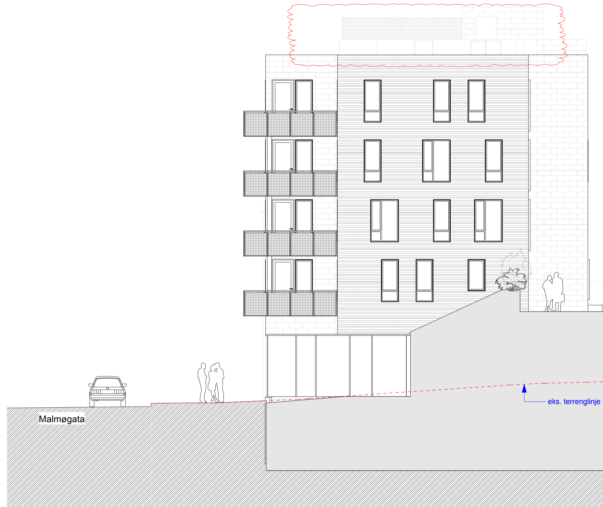
Fasade Syd Øst _Bygg A 1:100
